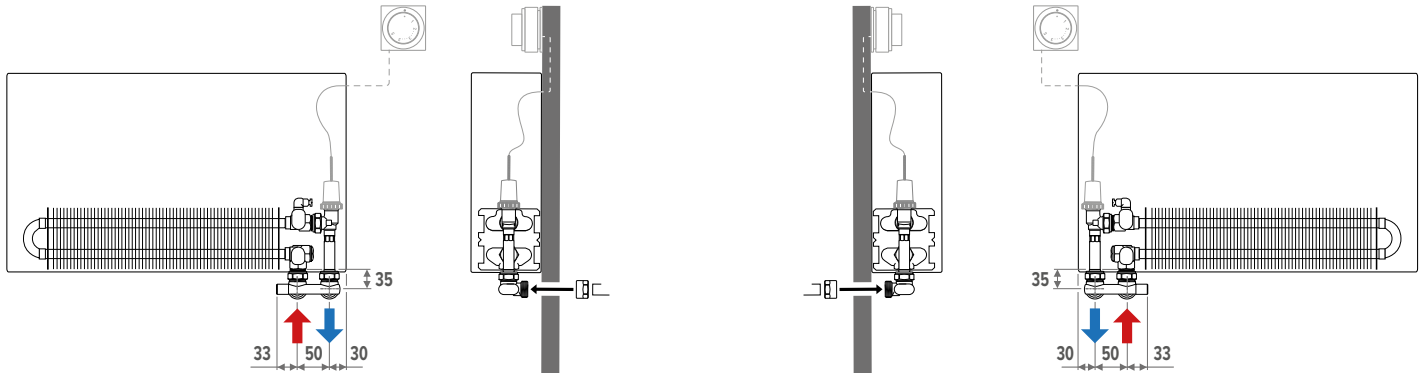
Ejemplo de conexión a la derecha (estándar)
