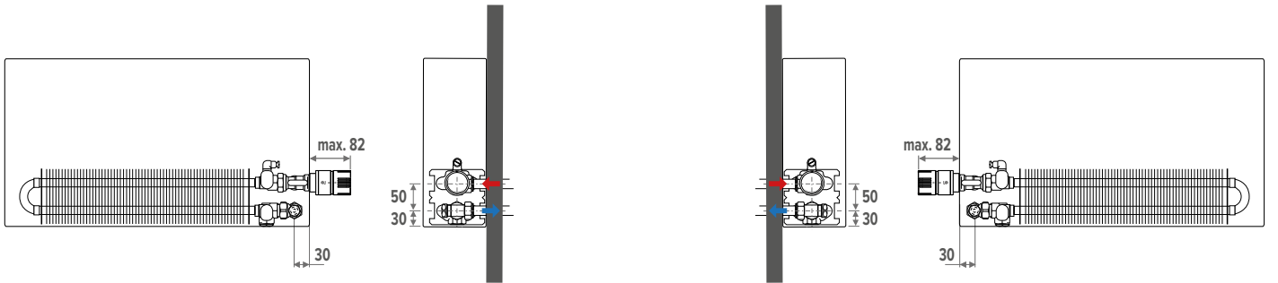
Ejemplo de conexión a la derecha (estándar)
