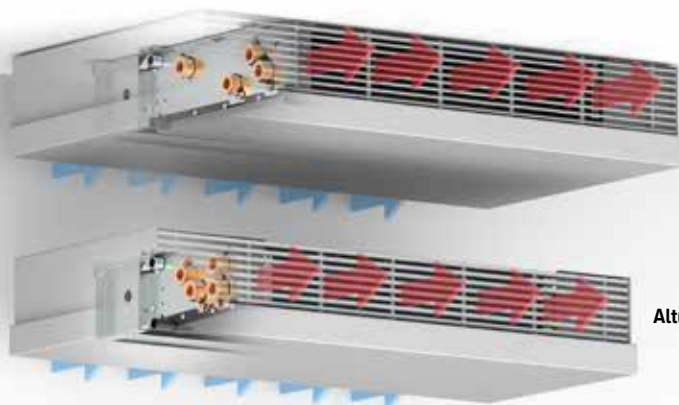
Altura 055 4 tubos
