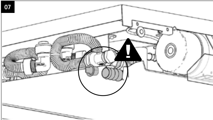
Niet-condenserend koelen - sluit de afvoernippel van de condensopvang af (Ø2cm).
