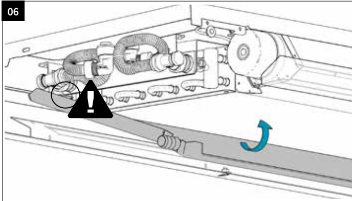
Plaats de condensopvang.
