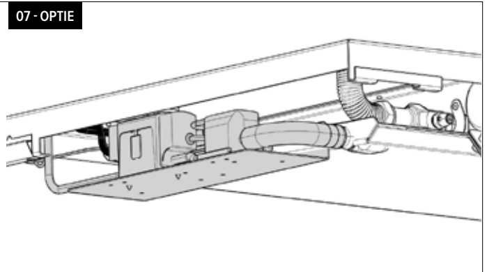
Condenserend koelen - voorgemonteerde condenspomp met onderbrekings contact (klasse I toestel).
