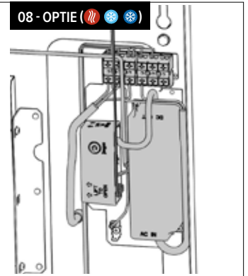
Aansluiting 230 VAC met waterdichte voeding en voorgemonteerde condenspomp met onderbrekings contact (klasse I toestel).
