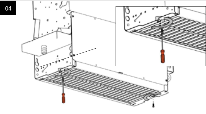
Fermez les verrous sur le côté de l'appareil et remplacez la vis.
