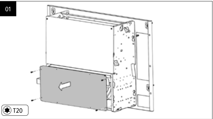
Dévissez les 4 vis du panneau avant inférieur et retirez ce panneau.
