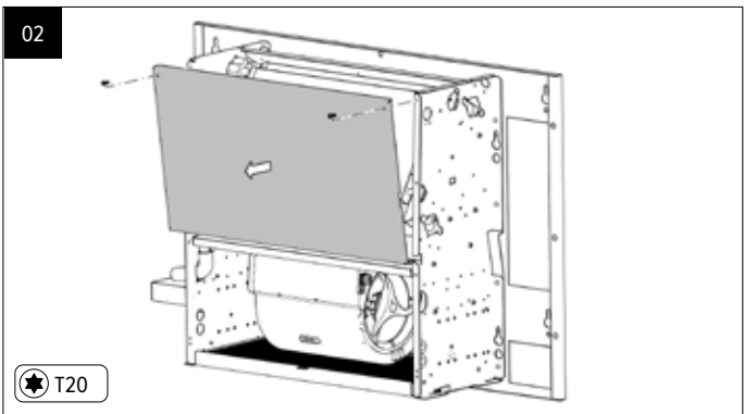
Retirez les 2 vis du panneau avant supérieur et ôtez-le.
