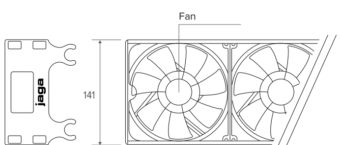
FAN UNIT (in mm)
