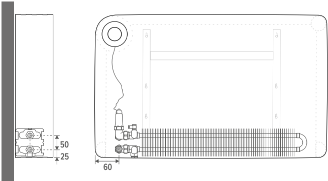
Ejemplo de conexión a la izquierda
