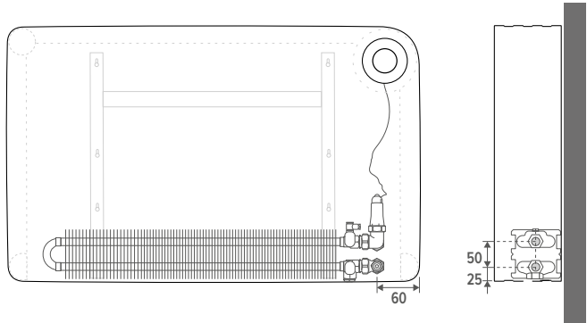
Ejemplo de conexión a la derecha (estándar)
