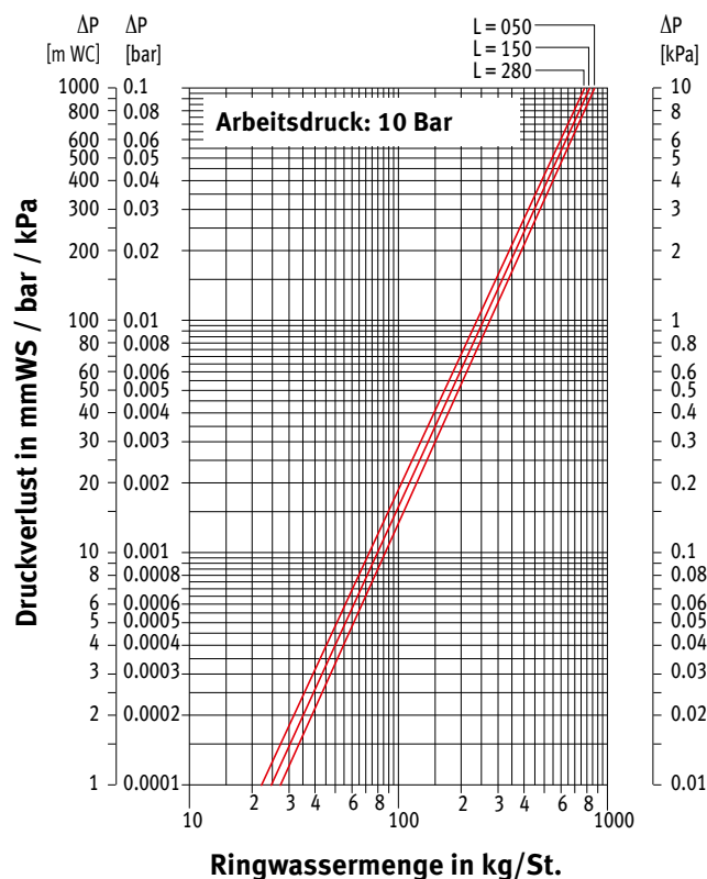
DRUCKVERLUSTE TYP 16
