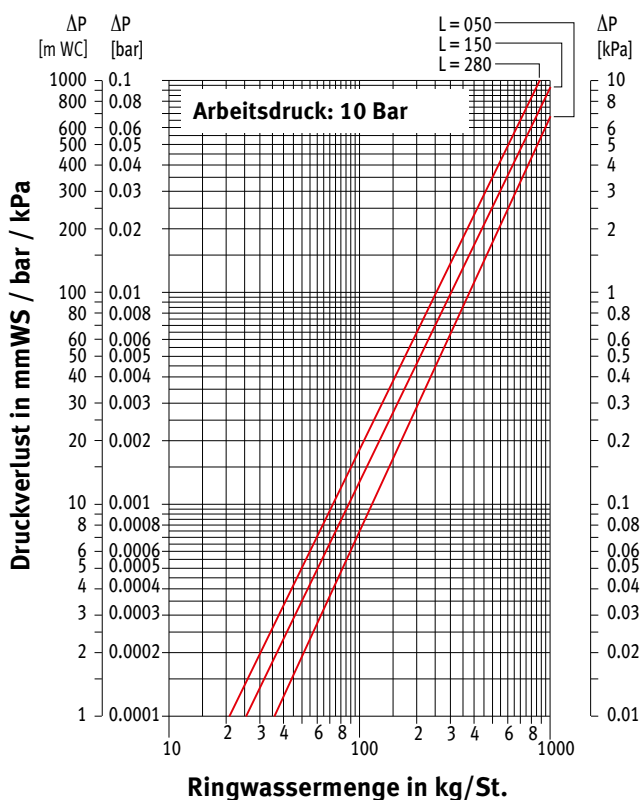
DRUCKVERLUSTE TYP 11
