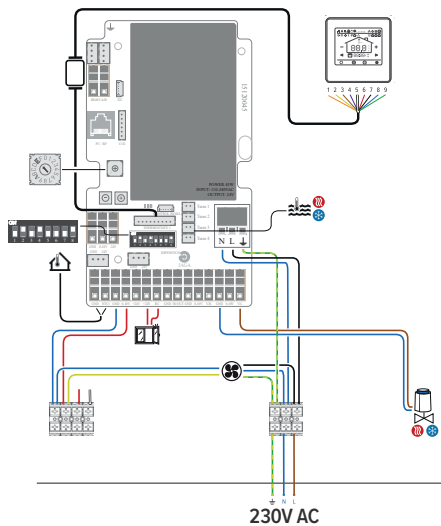
2-ROHR
