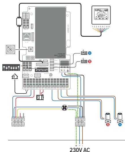
4-PIJP
