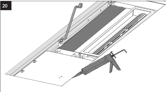
Fijnafstelling tot max. 0,8 cm voor een perfecte uitlijning met de afgewerkte vloer. Werk rondom af.
