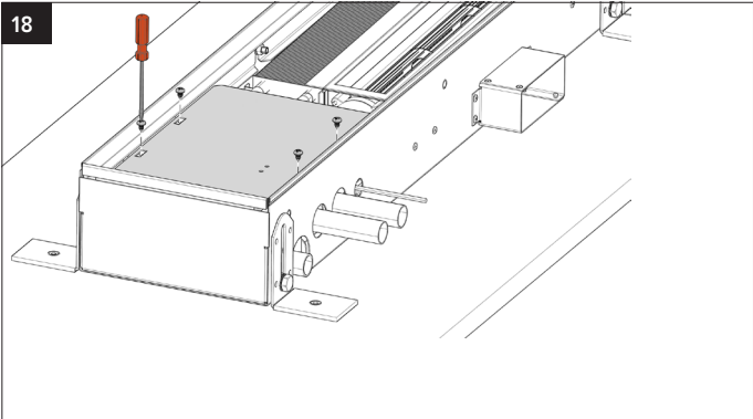
Monteer de ventiel afdekplaat. Dek de behuizing af met de beschermfolie en het werfpaneel.
