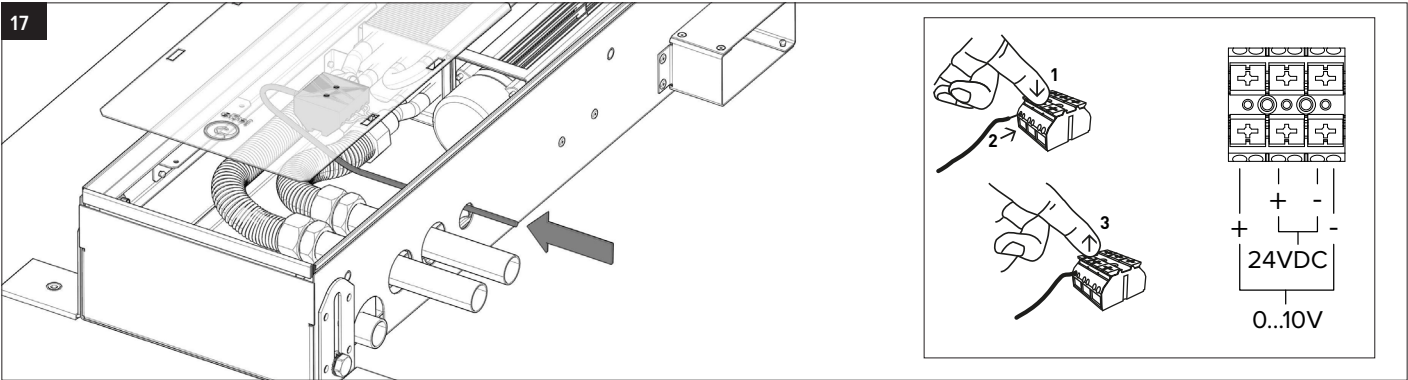
Aan de kant van de waterzijdige aansluiting bevindt zich ook het aansluitblokje voor de elektrische aansluiting. De elektrische aansluiting wordt aangesloten op het zwarte blokje dat aan de onderkant van de afdekplaat zit.
