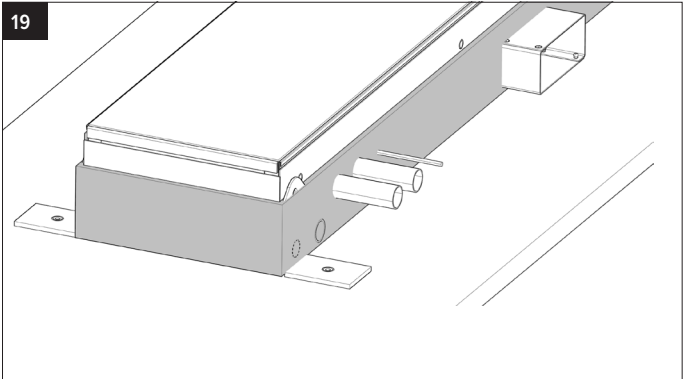
Als er een afwerkvloer wordt toegepast moet er randisolatie worden geplaatst rondom het volledige toestel, om het toestel te beschermen tegen spanningsverschillen.
